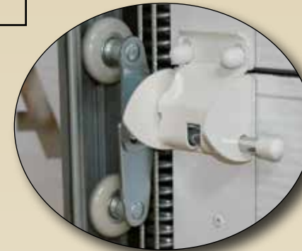
Charnière d'extrémité avec axe sur bague téflon Finition sublime + Roulette Téflon Tandem
